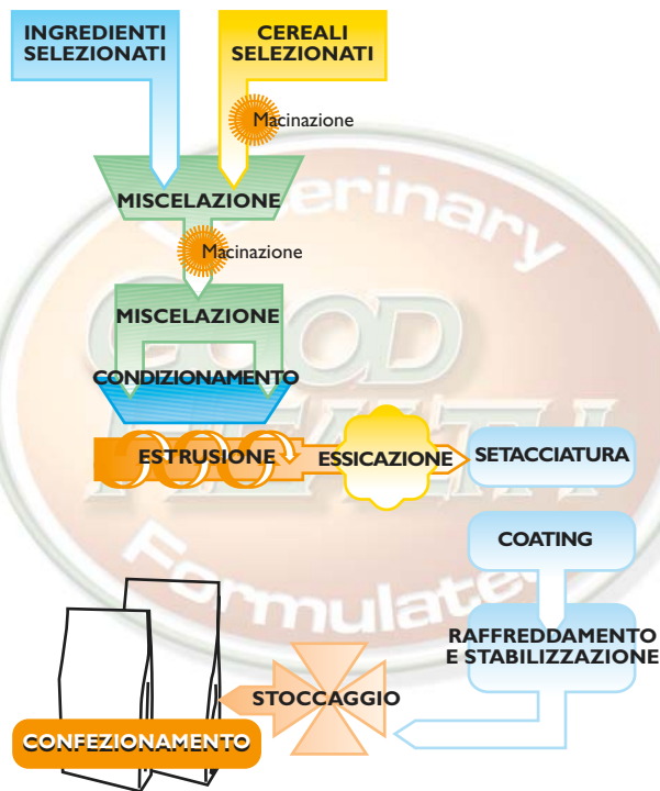
Flow-chart del PROCESSO PRODUTTIVO di estrusione
